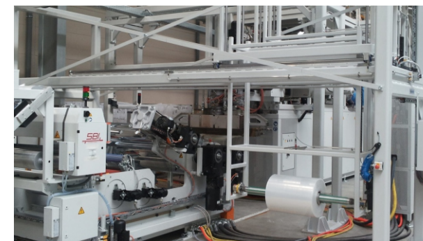
Hubabrollung, hier kann alles vom Boden aus bedient werden
