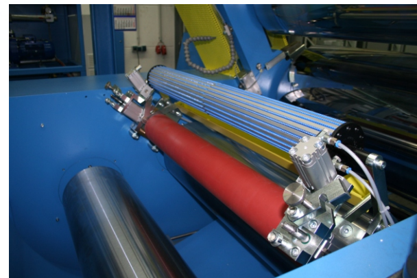
Laminierung eingebaut ins Glättwerk
